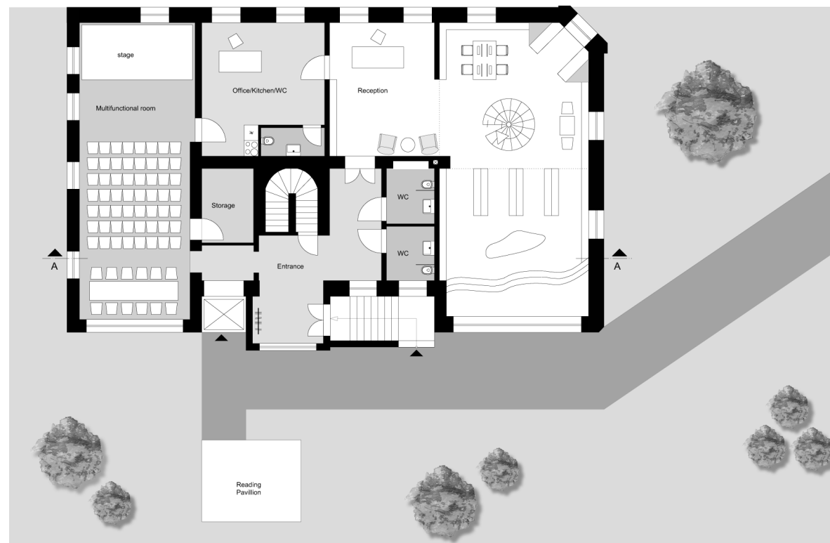
Studie dispozičního řešení v Místní knihovně ve Vranově nad Dyjí Autoři: Žiga Kodelič, Corinna Heller, Anna-Katharina Mathieu, ing. arch. Jan Kratochvíl
