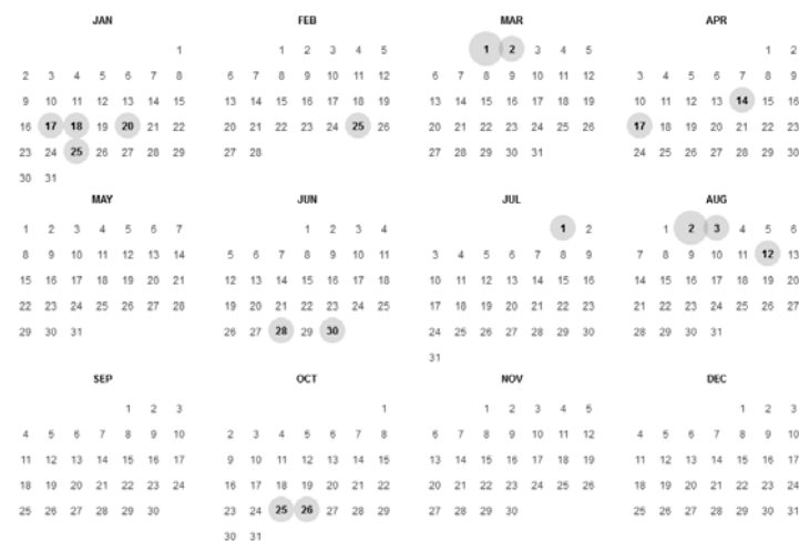
Obr. 4: Aplikace OpenWayback
